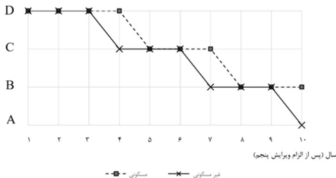
شکل ۱۹-۲-۱: زمان‌بندی الزام دستیابی به رده بازدهی انرژی در ساختمان‌های جدیدالاحداث
